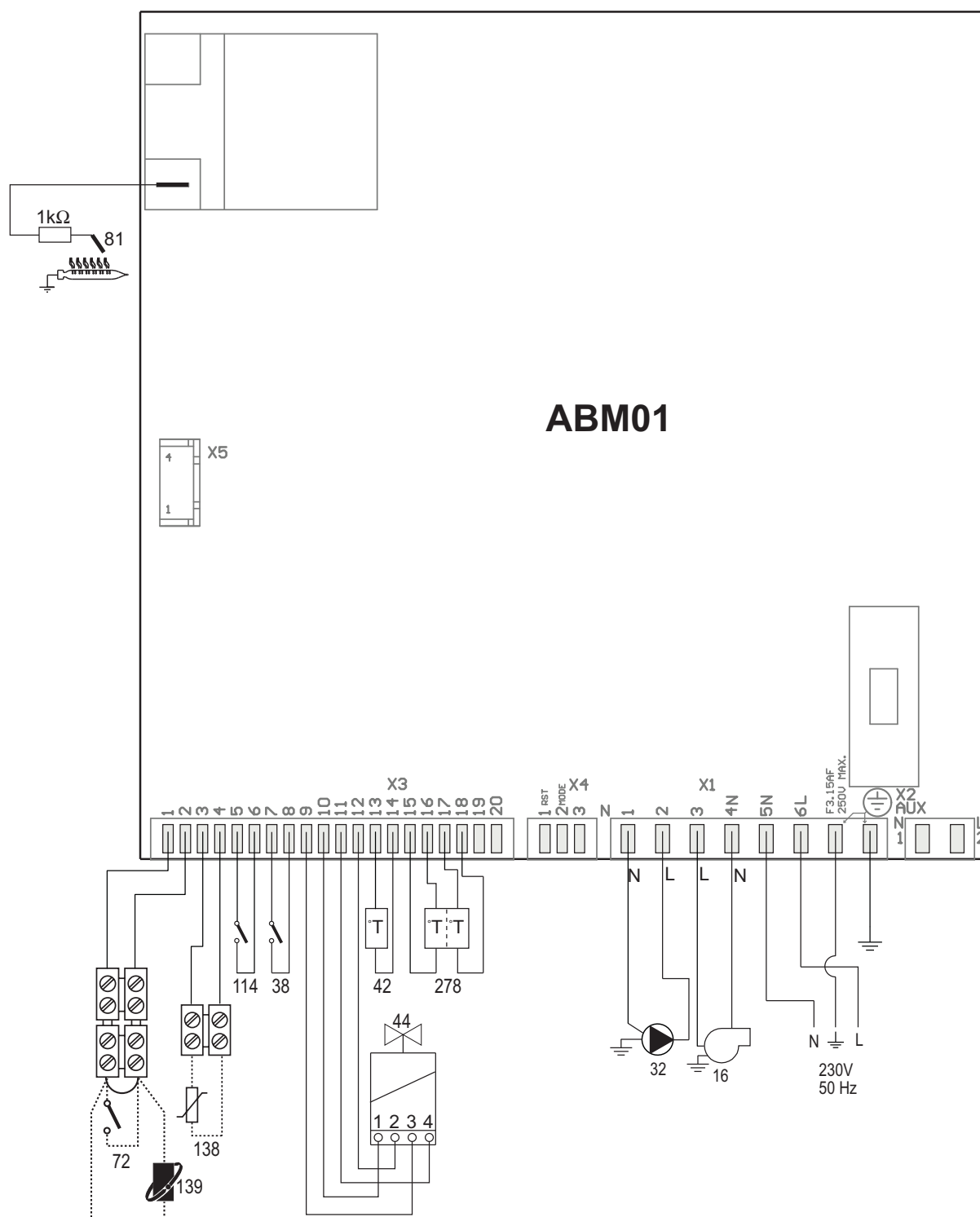
fig. 29 - Circuito elettrico
