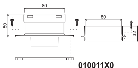
fig. 15 - Accessorio di partenza per condotti separati
