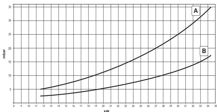
fig. 26 - Diagramma pressione - potenza (FOX D 32 S)
