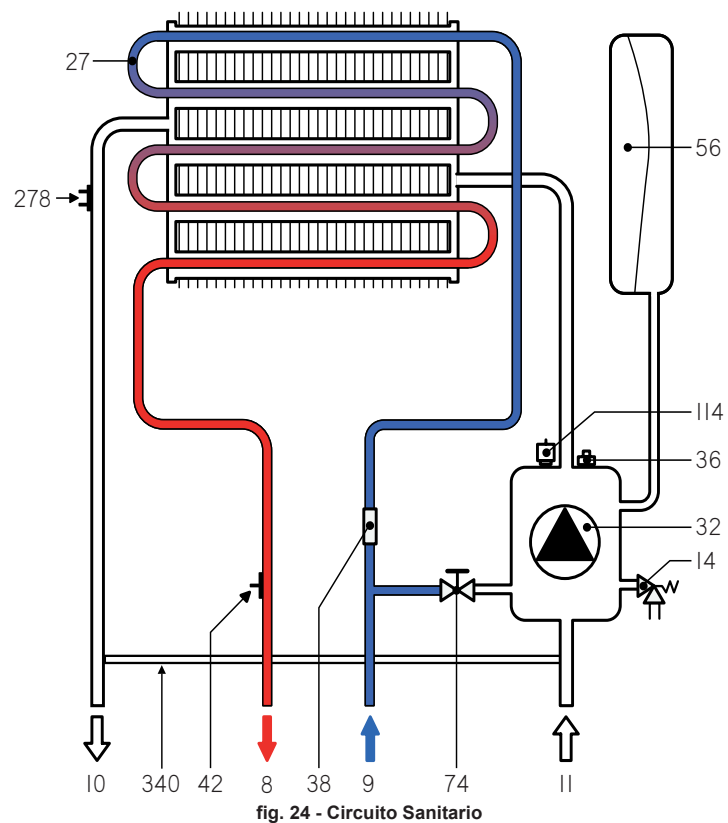
fig. 24 - Circuito Sanitario
