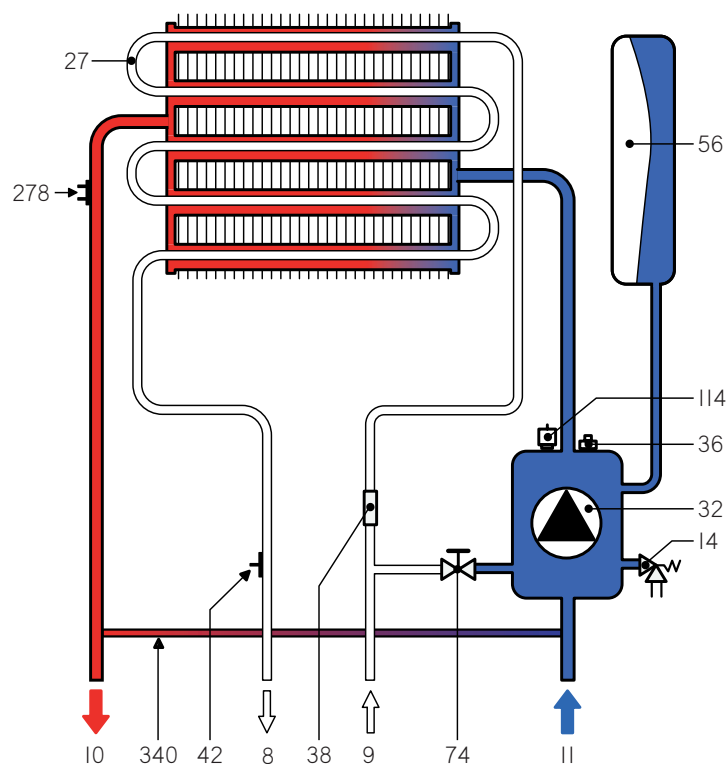
fig. 23 - Circuito Riscaldamento
