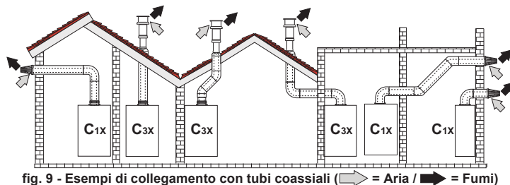
fig. 9 - Esempi di collegamento con tubi coassiali (⇐ = Aria / ⇨ = Fumi)
