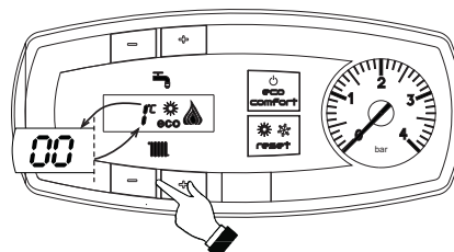
fig. 17 - Modalità TEST (potenza riscaldamento = 100%)
