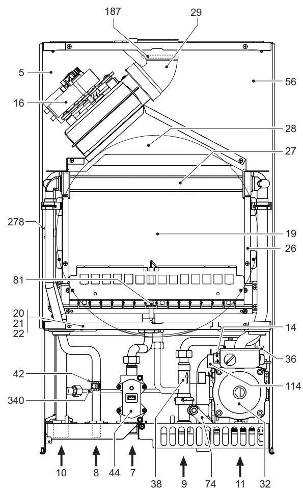
fig. 22 - Vista generale FOX D 32 S
